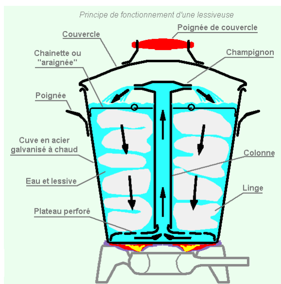
Figure 1. Schéma de fonctionnement d'une lessiveuse
